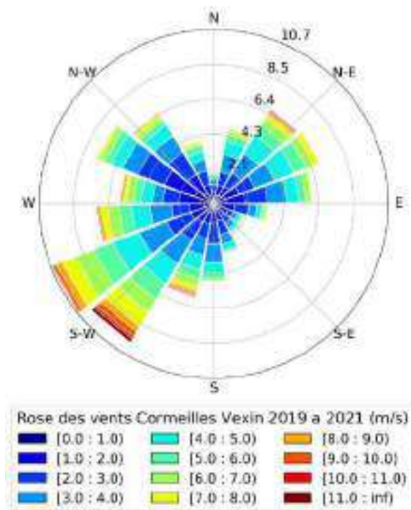
Figure 38 : Rose des vents à la station de Corneilles en Vexin, période 2019-2021
